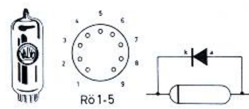
ANSCHLÜSSE DER VALVO-RÖHREN
